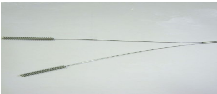
Róždźki dwuramiennie. Rys. Nr 9
